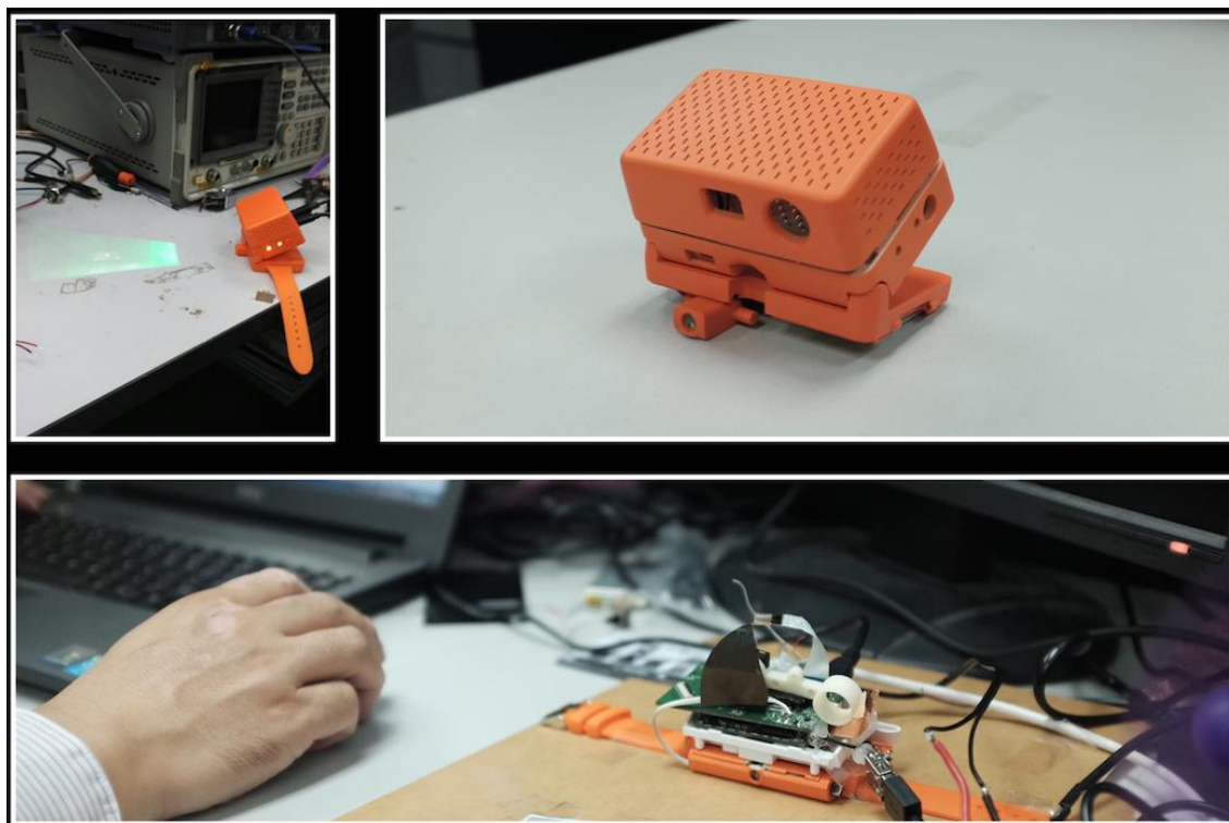
图 4 Cicret2016 年公布的最新研发进展
