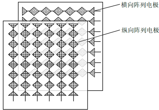
图 8 触摸屏电容式触摸感应例，感应线必须是“纵横交错”
